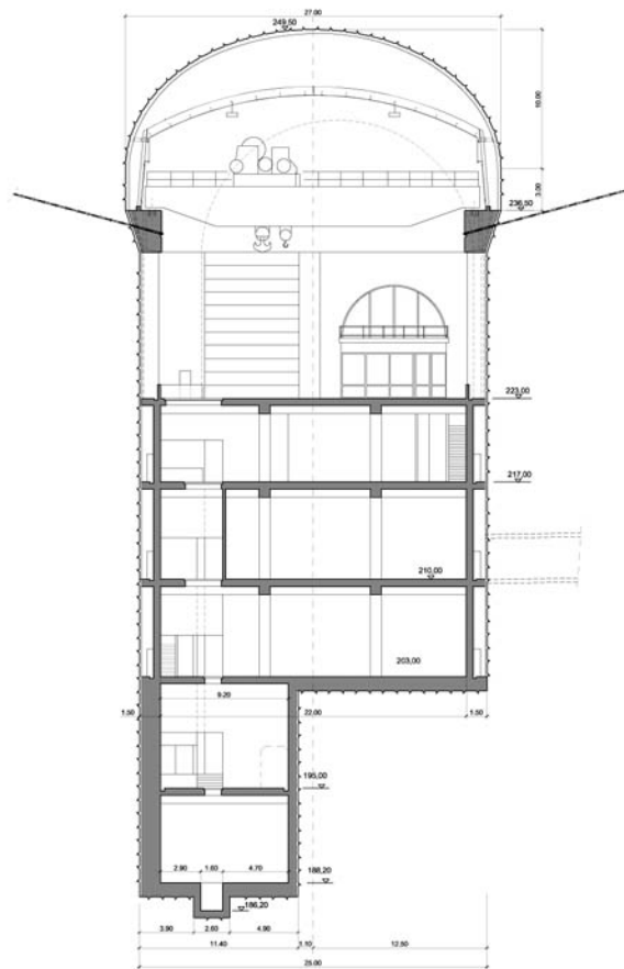
CORTE C-C
