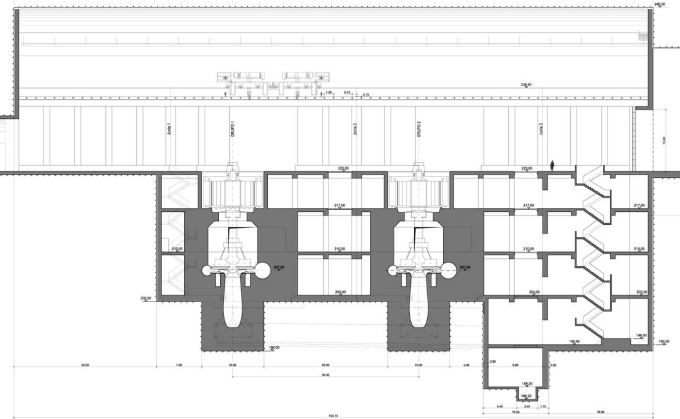
CORTE LONGITUDINAL A-A
