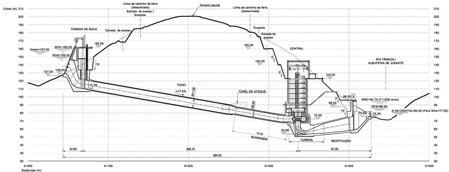
PERFIL LONGITUDINAL PELO EIXO DO CIRCUITO HIDRÁULICO
