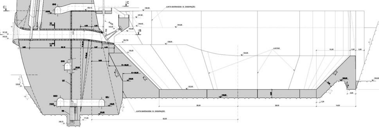
CORTE PELO EIXO DA DESCARGA DE FUNDO
